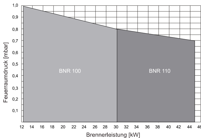
Abb. 25: Leistungsdiagramm
