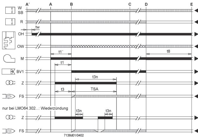
Abb. 19: Programmablauf LMO 44
