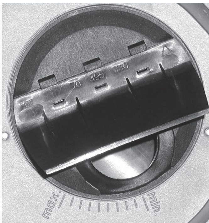
Abb. 13: Lufteinlaufdüse und Skala
