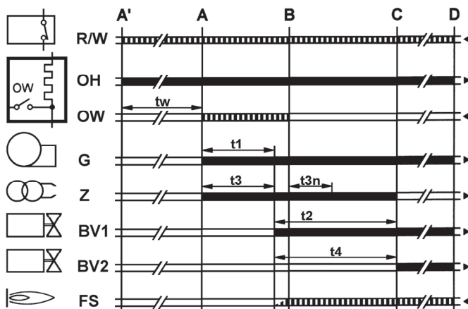
Abb. 20: Programmablauf LMO 64
