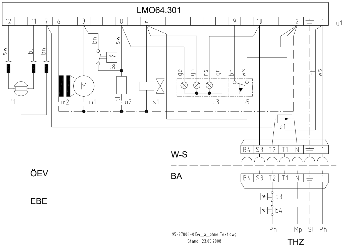
Abb. 10: Schaltplan für FA Siemens LMO 64 (mit Gebläsenachlauf)
