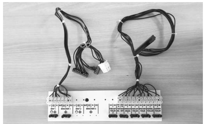
Abb. 30: Regler-Kabelbaum mit Klemmen und Steckverbinder zum Kesselschaftfeld.
