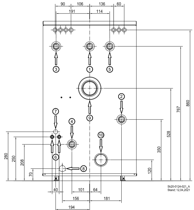
Abb. 3: Abmessungen Rückseite
