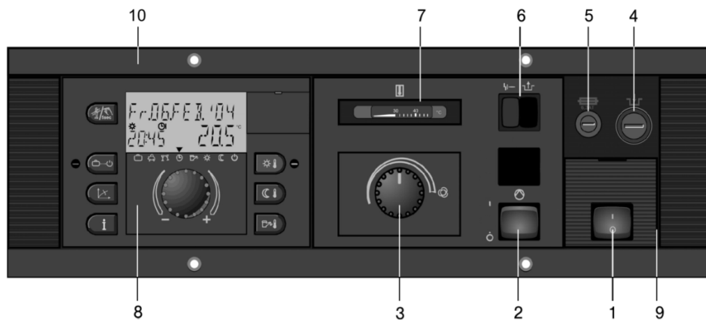
Abb. 101: Kesselschaltfeld ECOHEAT Plus...
