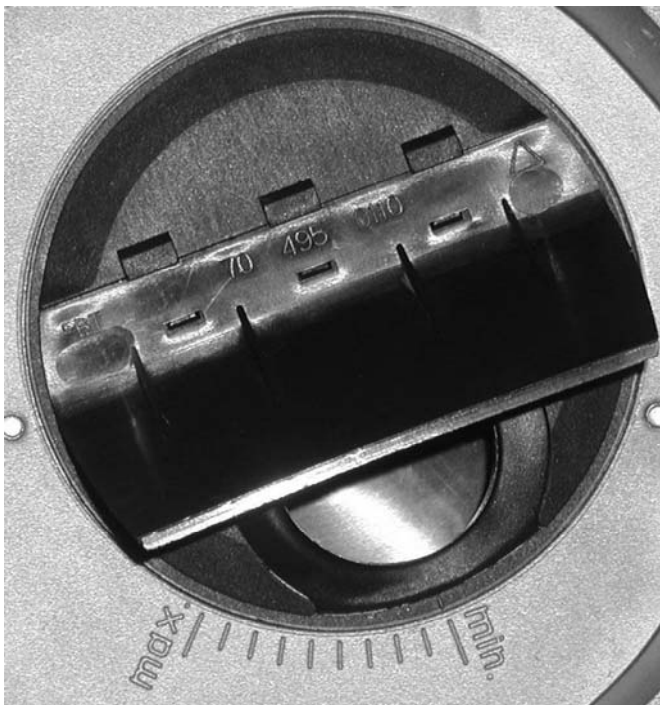
Abb. 73: Lufteinlaufdüse
