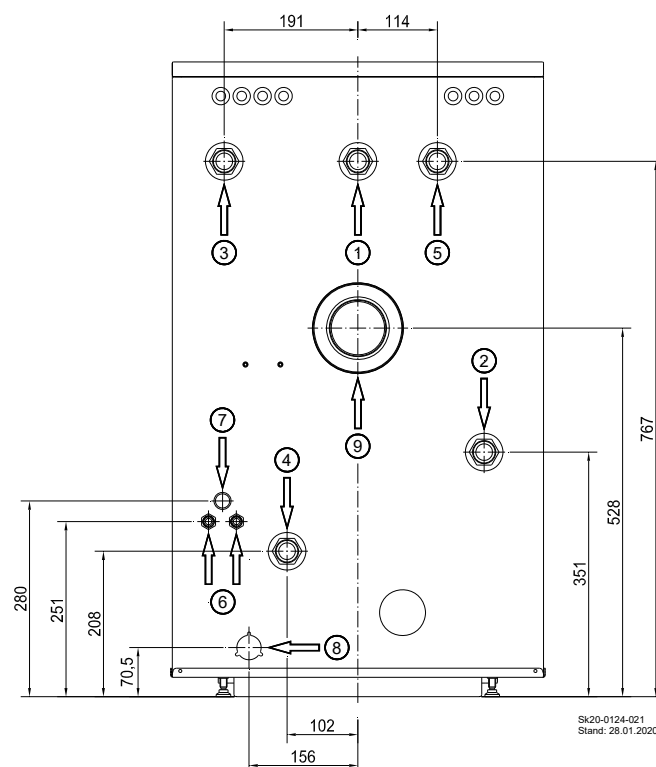
Abb. 20: Hydraulische Anschlüsse an der Kesselnückwand
