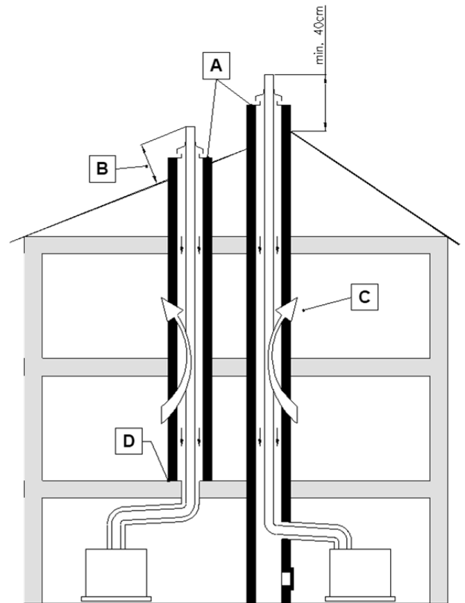
Abb. 41: Schachtqualität für Abgasleitungen
