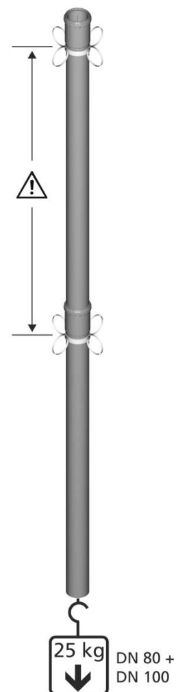
Abb. 55: Abgasrohre mit Stoppring-Technik ①
